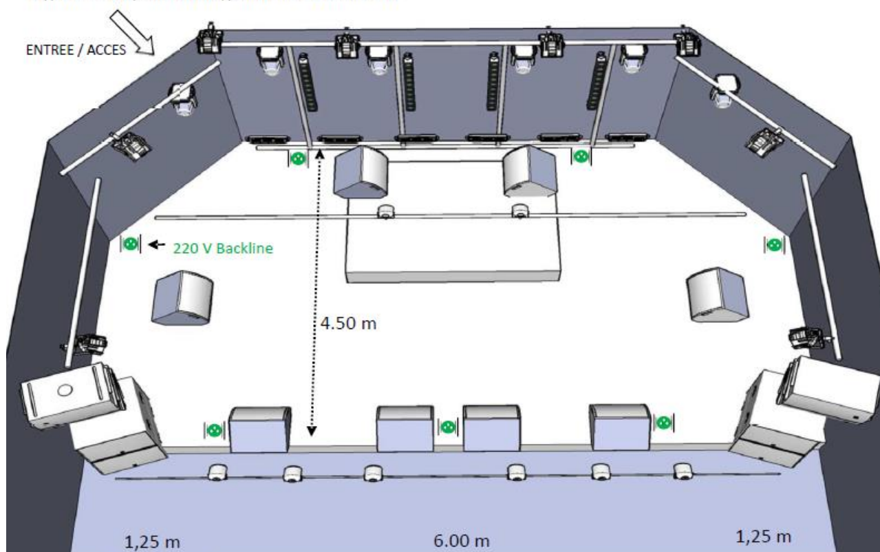
Figure 1. Implantation générale - vue dessus
