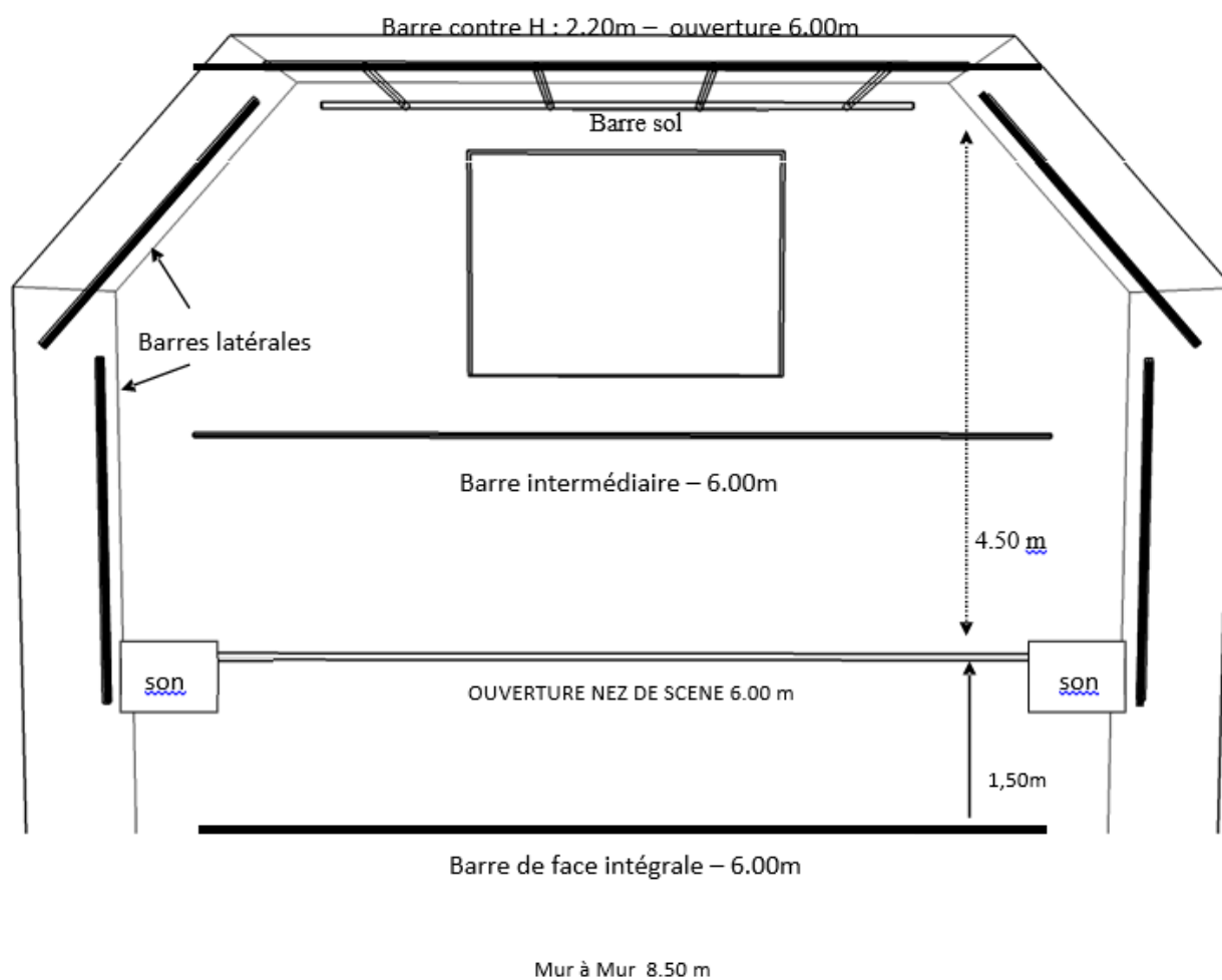
Figure 2. Gril - Détail des accroches
